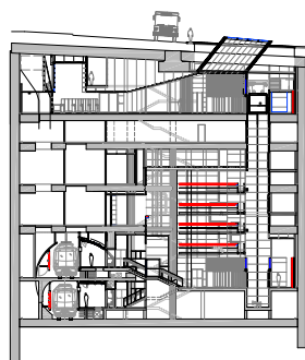
SECCIÓ DEL POU / SECCIÓ DEL POZO / WELLS SECTION
