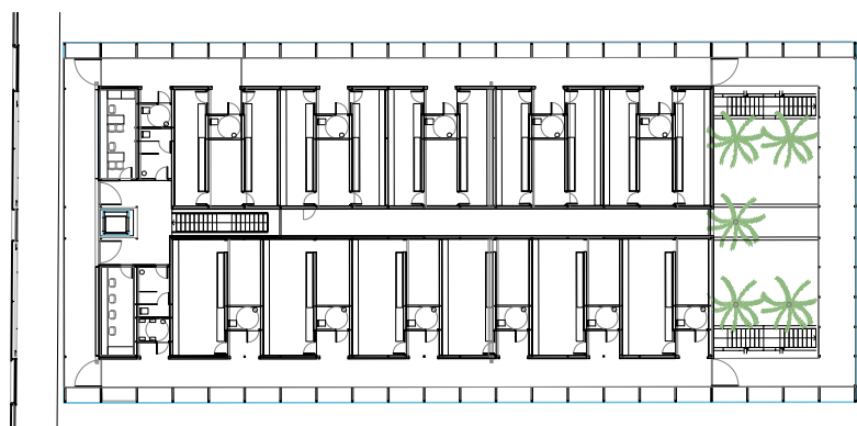
PLANTA D'ACCÉS / PLANTA DE ACCESO / ENTRANCE FLOOR
