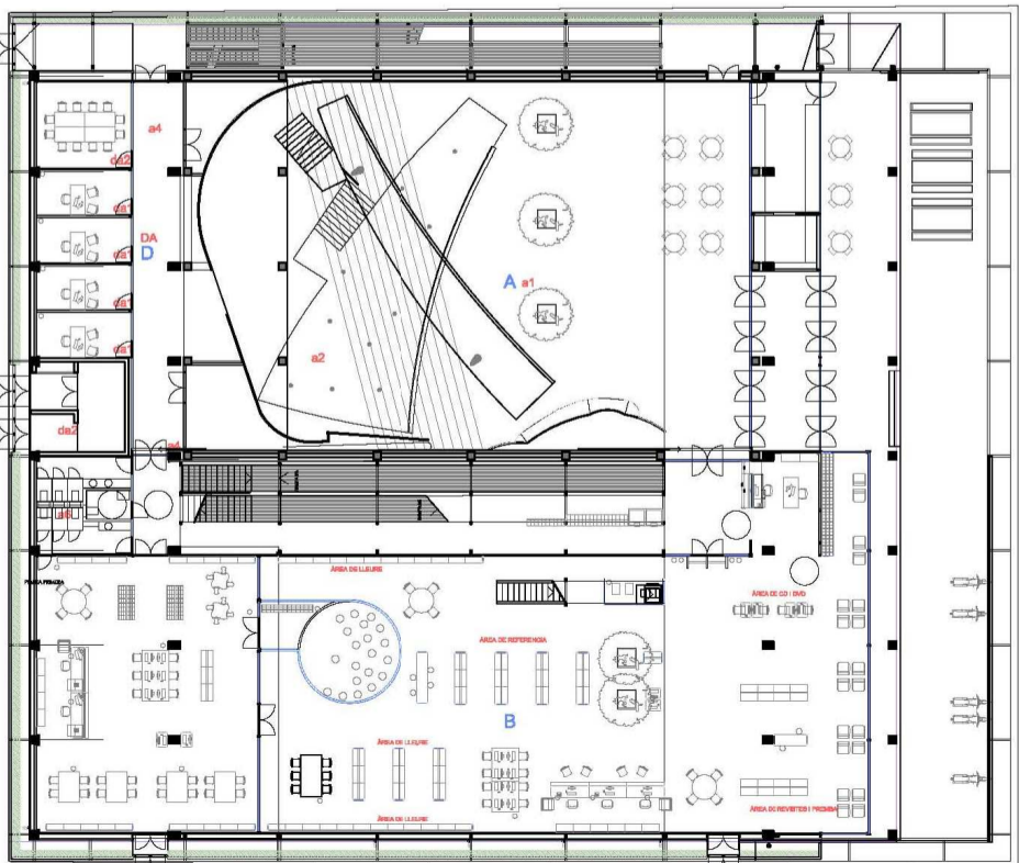
PLANTA BAIXA / PLANTA BAJA / GROUND FLOOR PLAN
