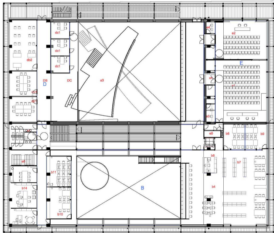
PLANTA PRIMERA / PLANTA PRIMERA / FIRST FLOOR PLAN
